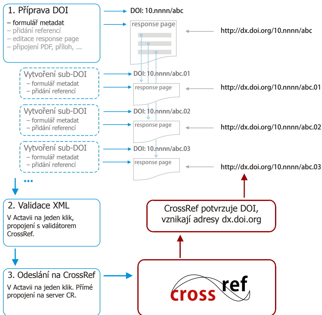
Schéma založení a zveřejnění DOI, modře Actavia, červeně CrossRef.
